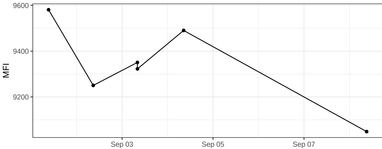
BUV737-A
