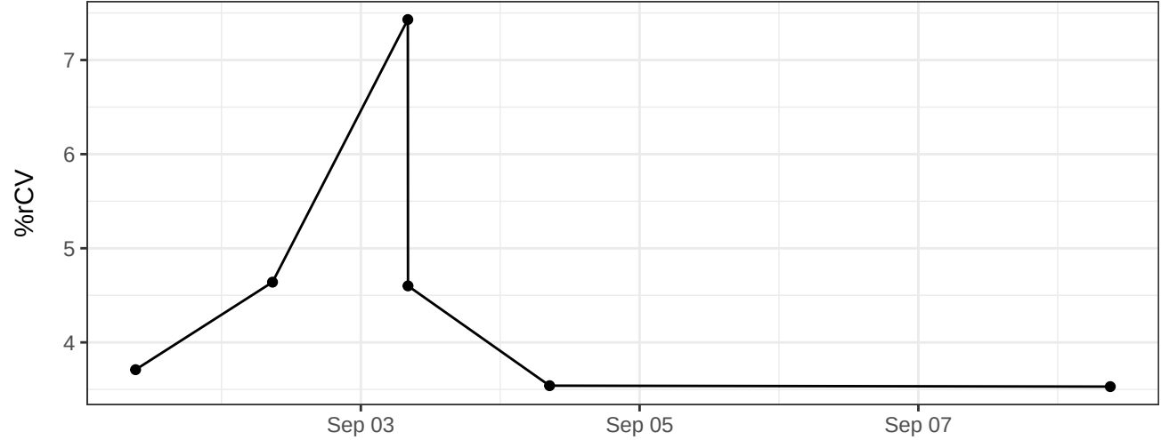
BUV805-A-% rCV
